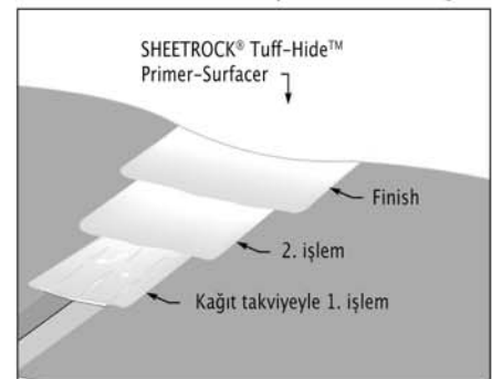
SHEETROCK® Tuff-Hide™ bir işlemden tasarruf sağlar
